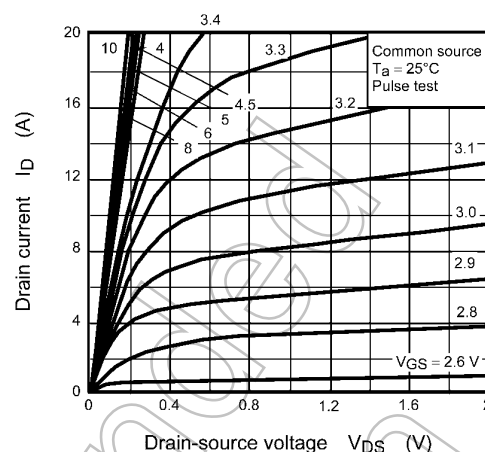
Fig. 8.2 I_D - V_{DS}
